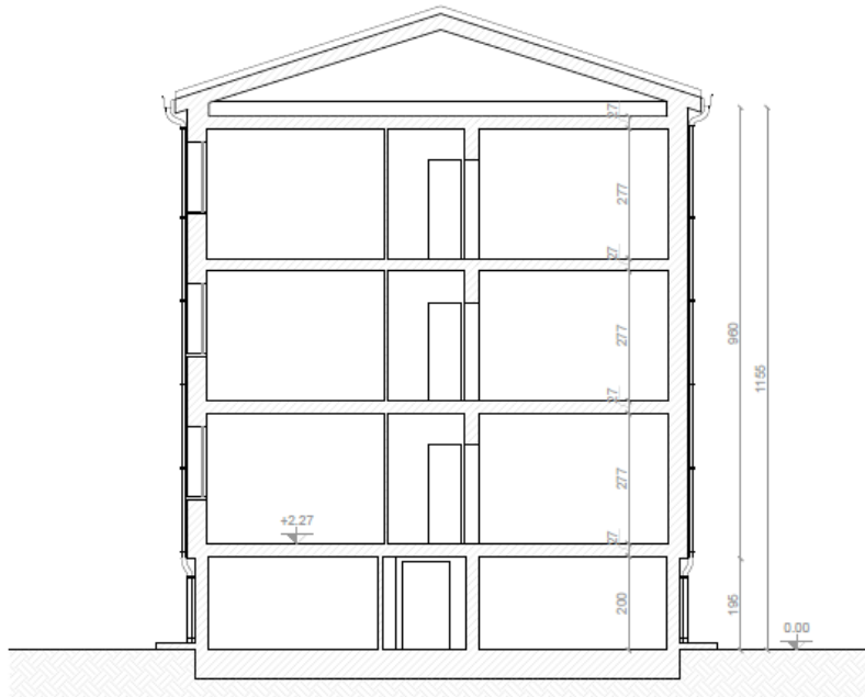
SEZIONE B-B
