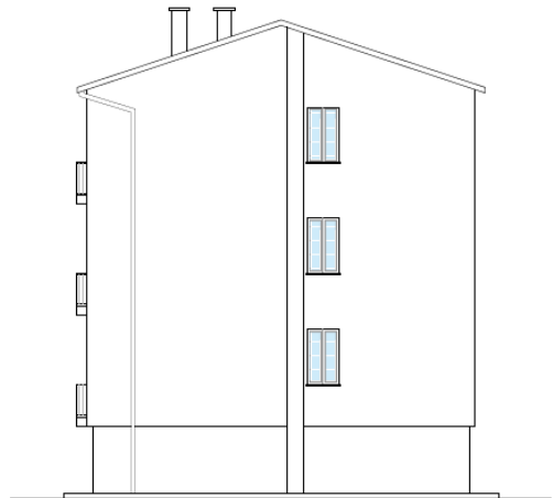
PROSPETTO NORD
