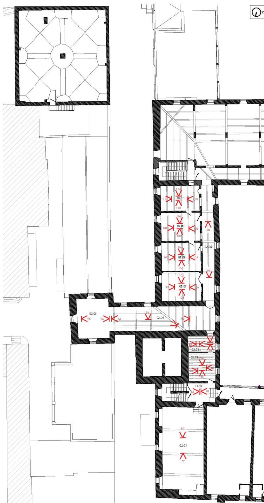
Figura 91 - Planimetria piano secondo, con indicazione dei coni ottici delle riprese fotografiche.
