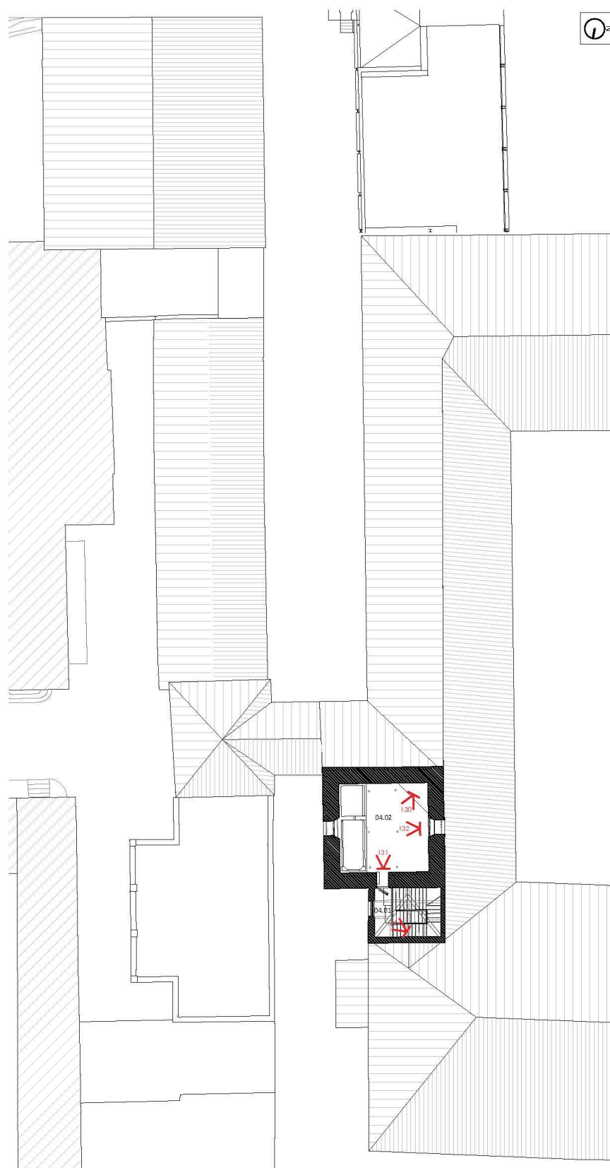
Figura 143 - Planimetria livello torre, con indicazione dei coni ottici delle riprese fotografiche.
