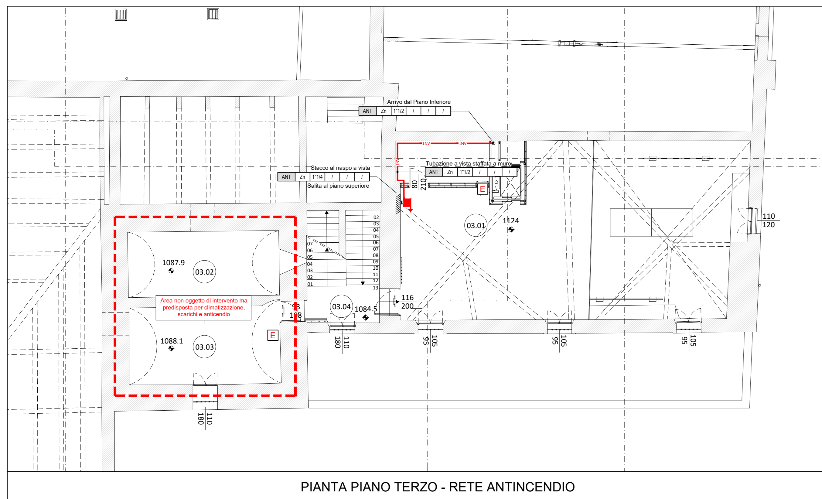
PIANTA PIANO TERZO - RETE ANTINCENDIO
