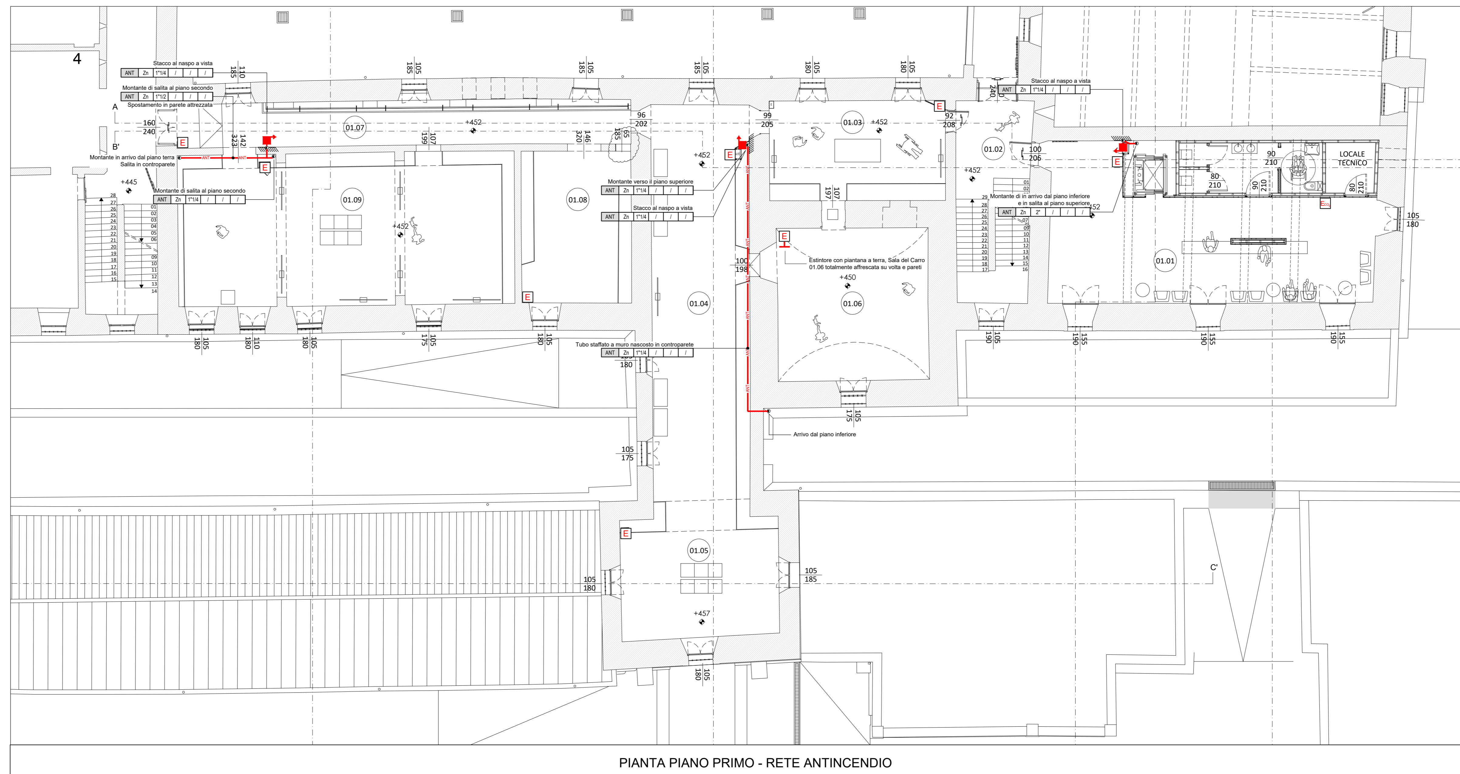
PIANTA PIANO PRIMO - RETE ANTINCENDIO
