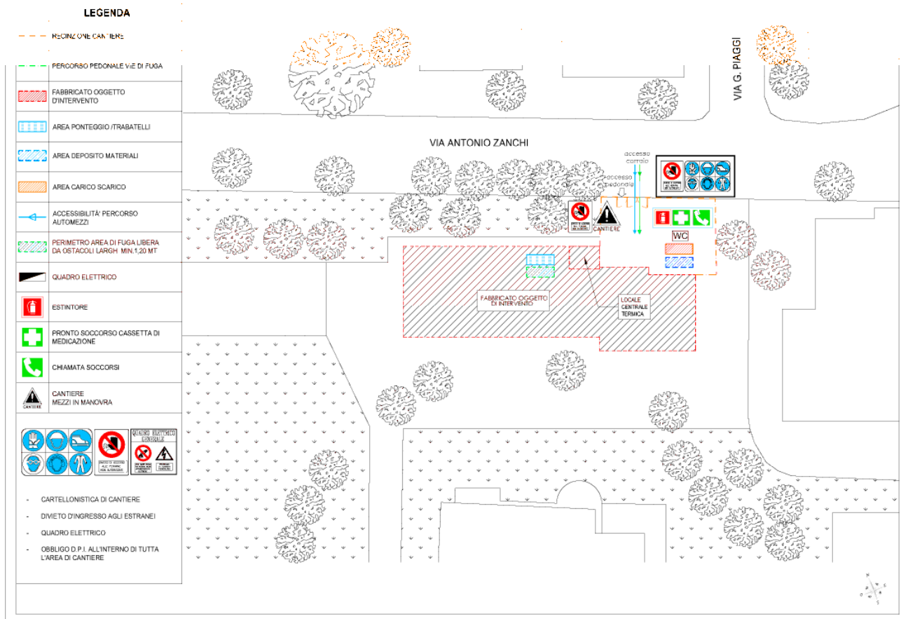
Figura 2 – Layout di cantiere –
