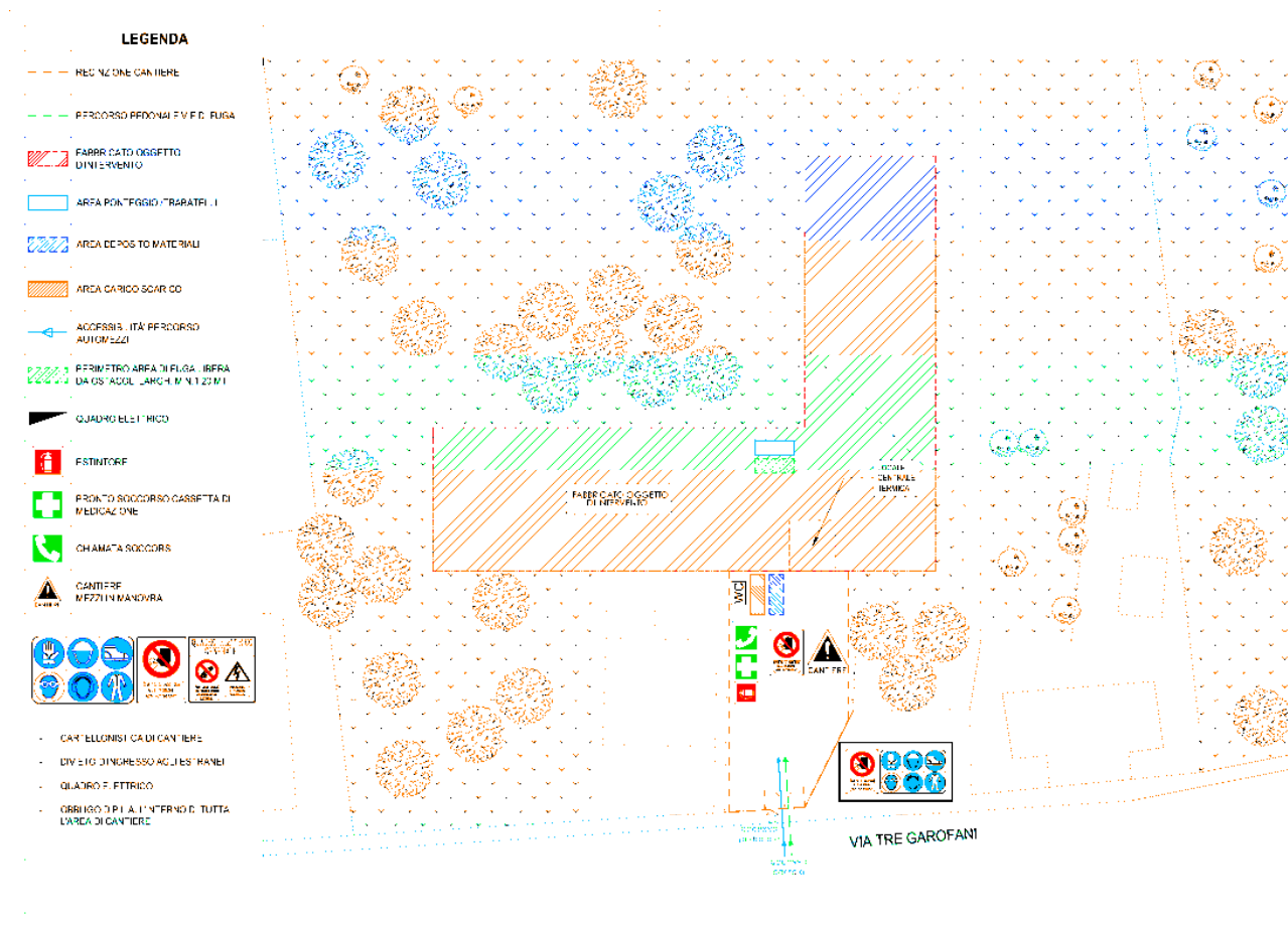
Figura 2 – Layout di cantiere –
