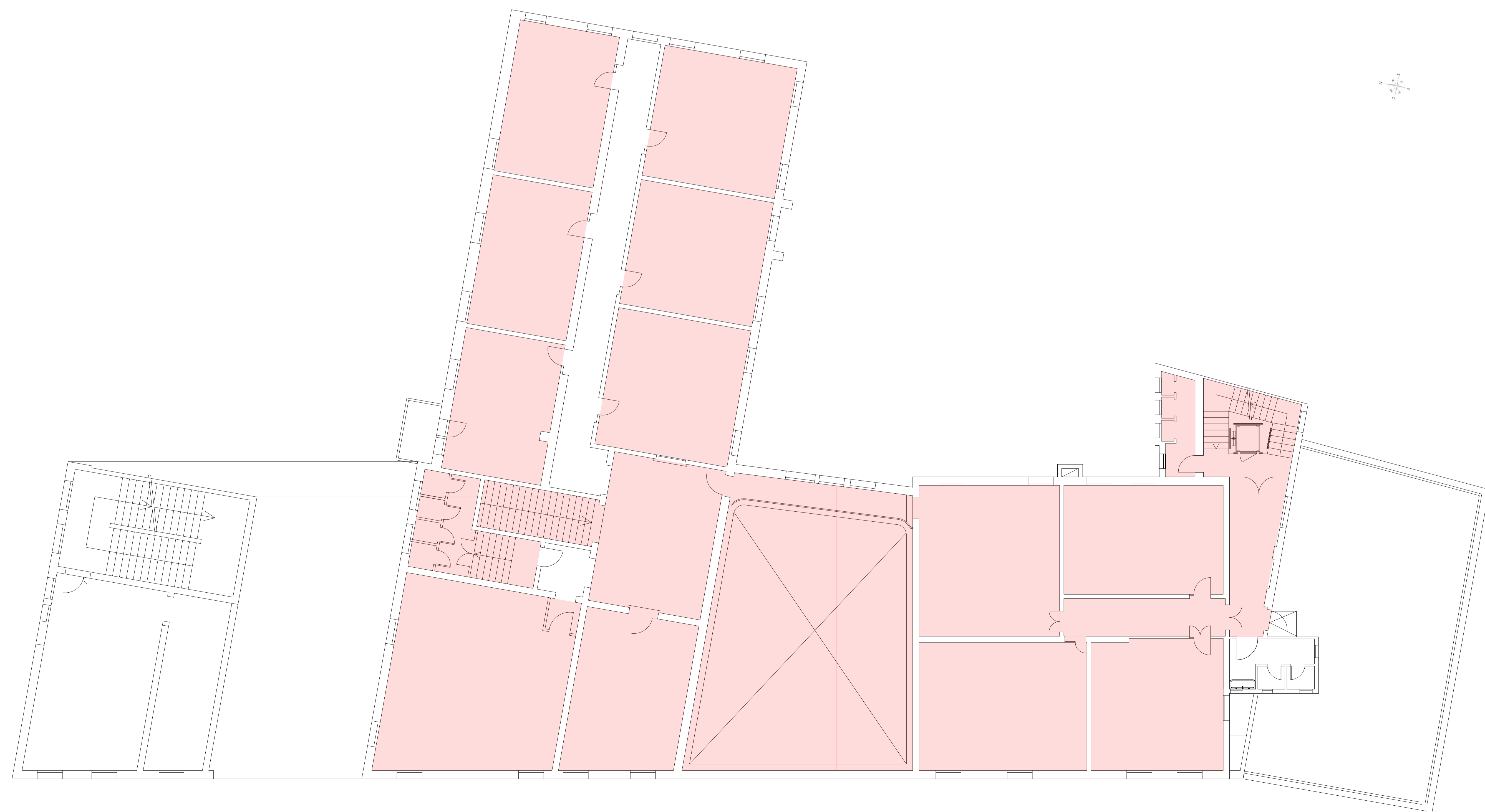
PIANTA PIANO SECONDO IMPIANTO DI RISCALDAMENTO SCALA 1:100
