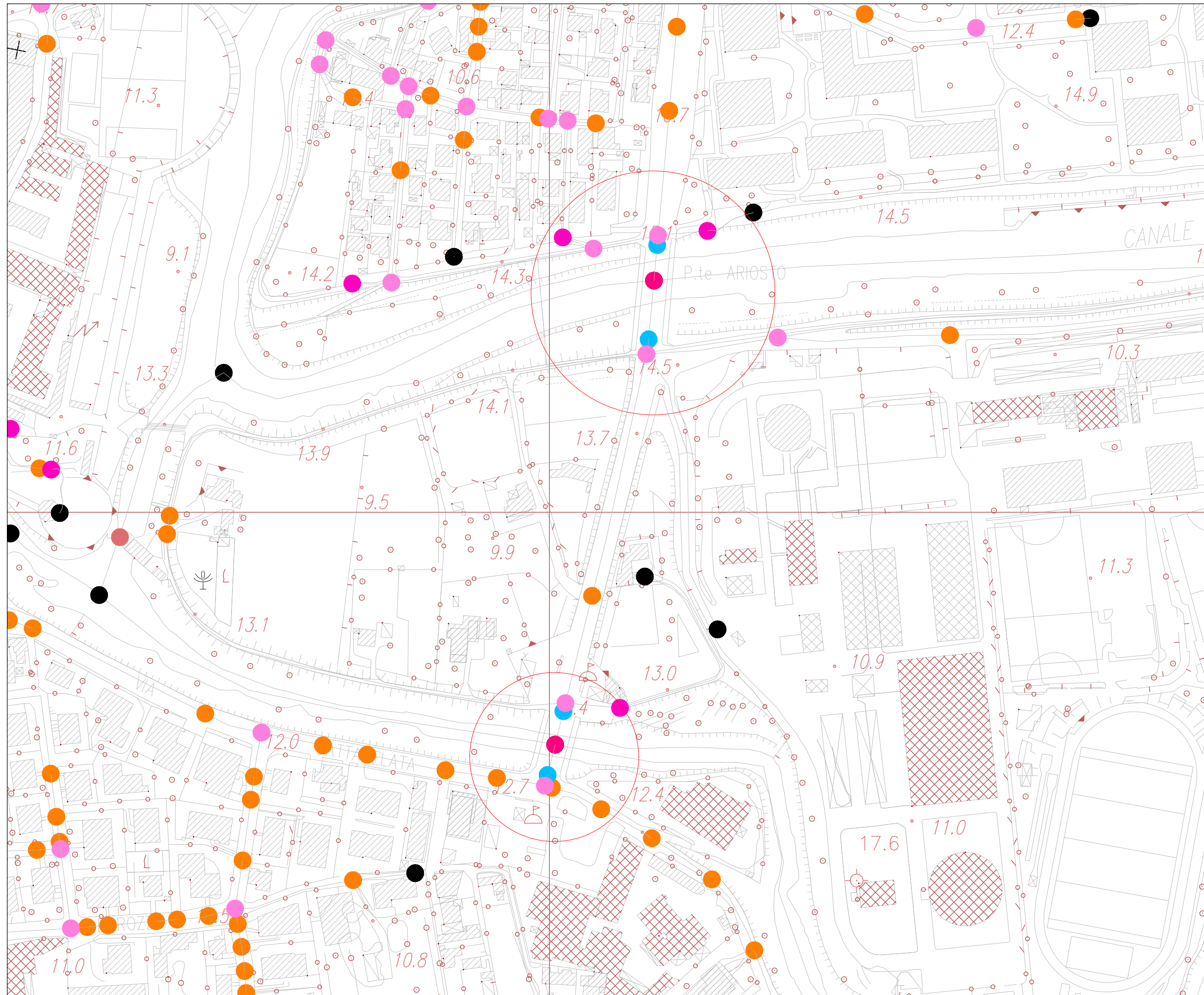
PLANIMETRIA GENERALE SU CTR SCALA 1:2000
