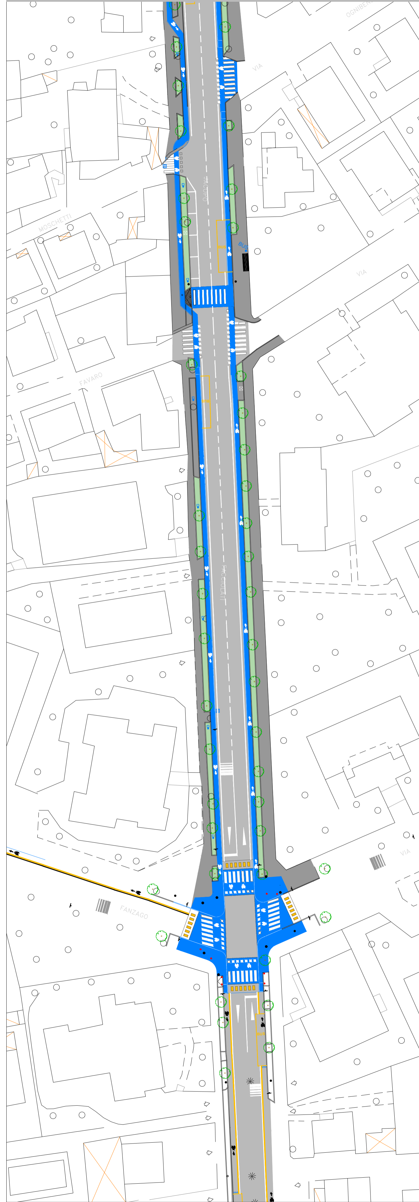
Stato di Fatto Planimetria Generale - 7° Tratto via Facciolati - Pontecorvo - scala 1:500
