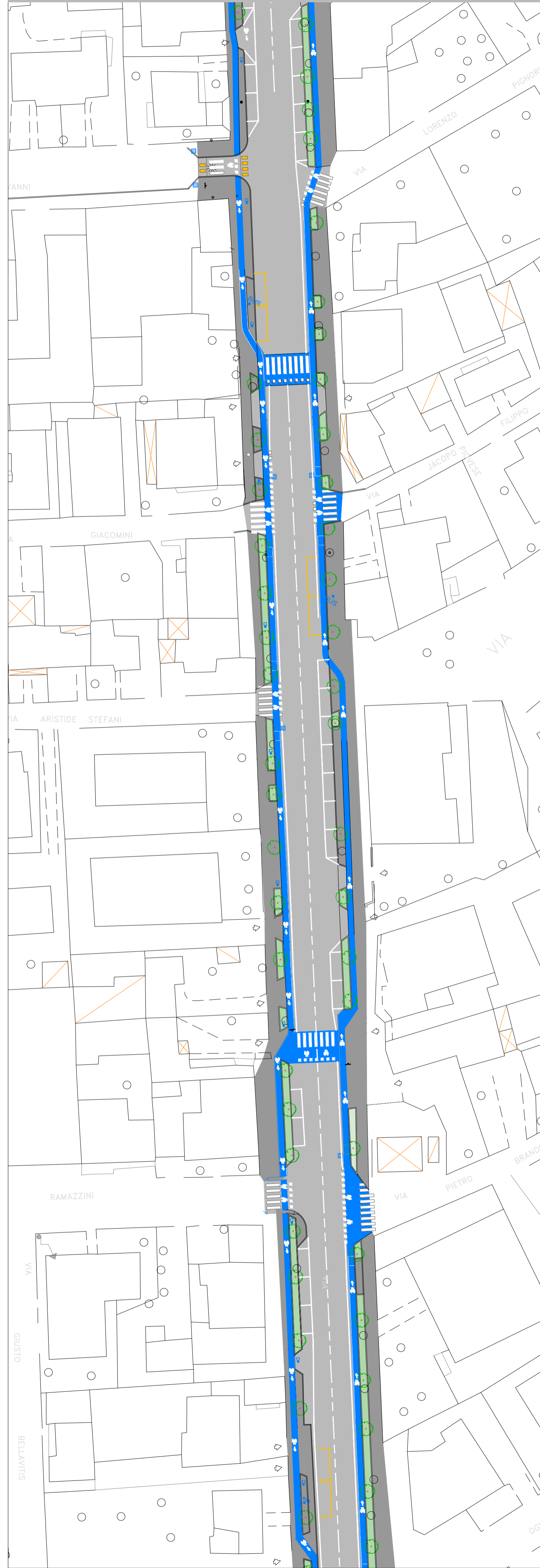
Stato di Fatto Planimetria Generale - 6° Tratto via Facciolati - Pontecorvo - scala 1:500
