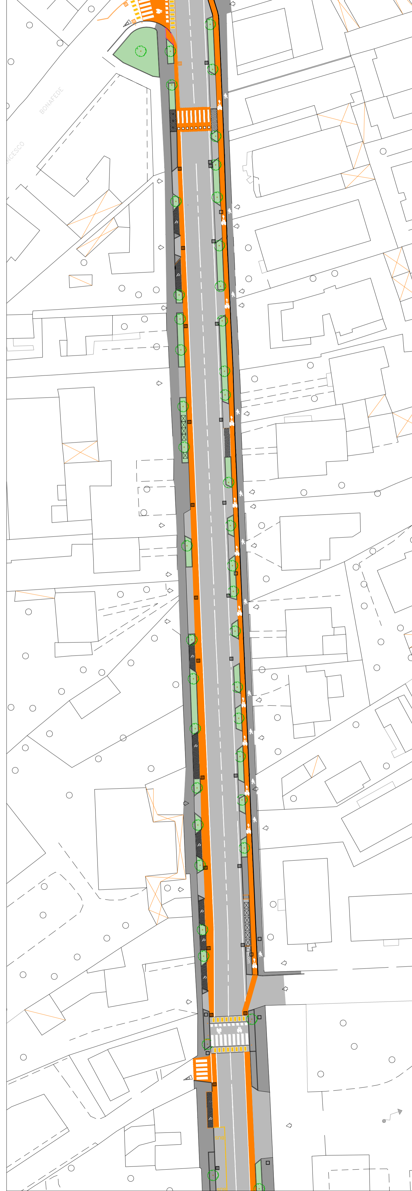
Stato di progetto Planimetria Generale - 4° Tratto via Facciolati - Pontecorvo - scala 1:500
