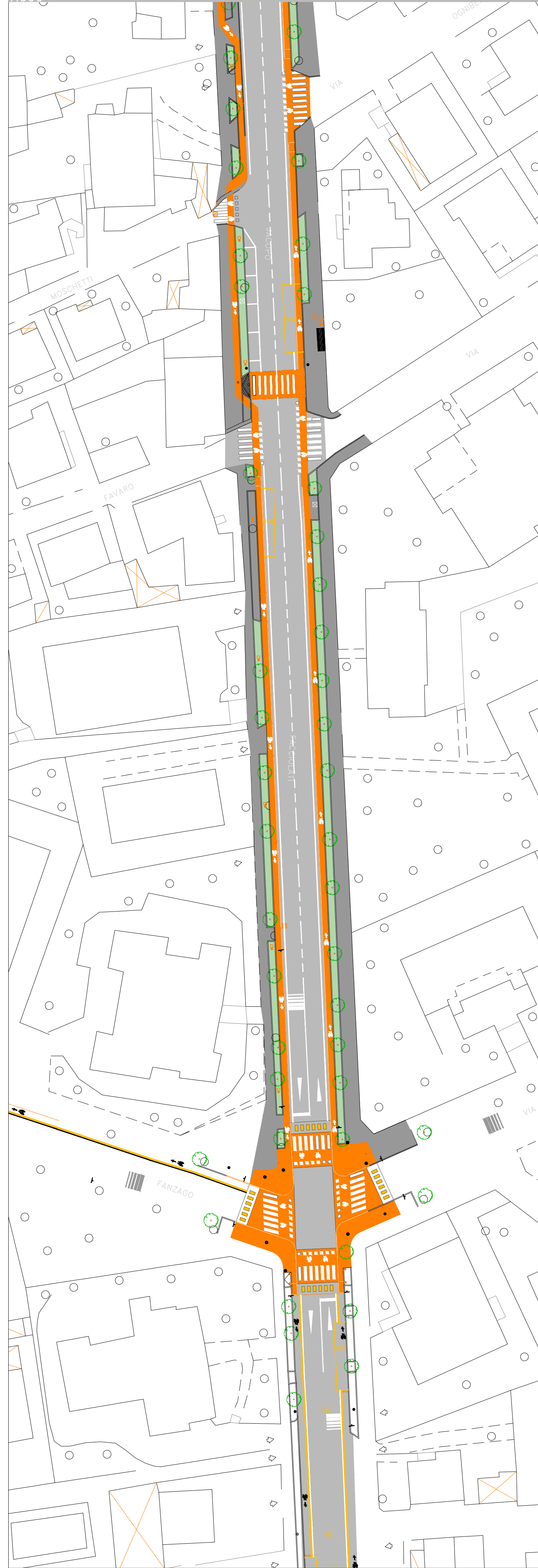
Stato di Progetto Planimetria Generale - 7° Tratto via Facciolati - Pontecorvo - scala 1:500
