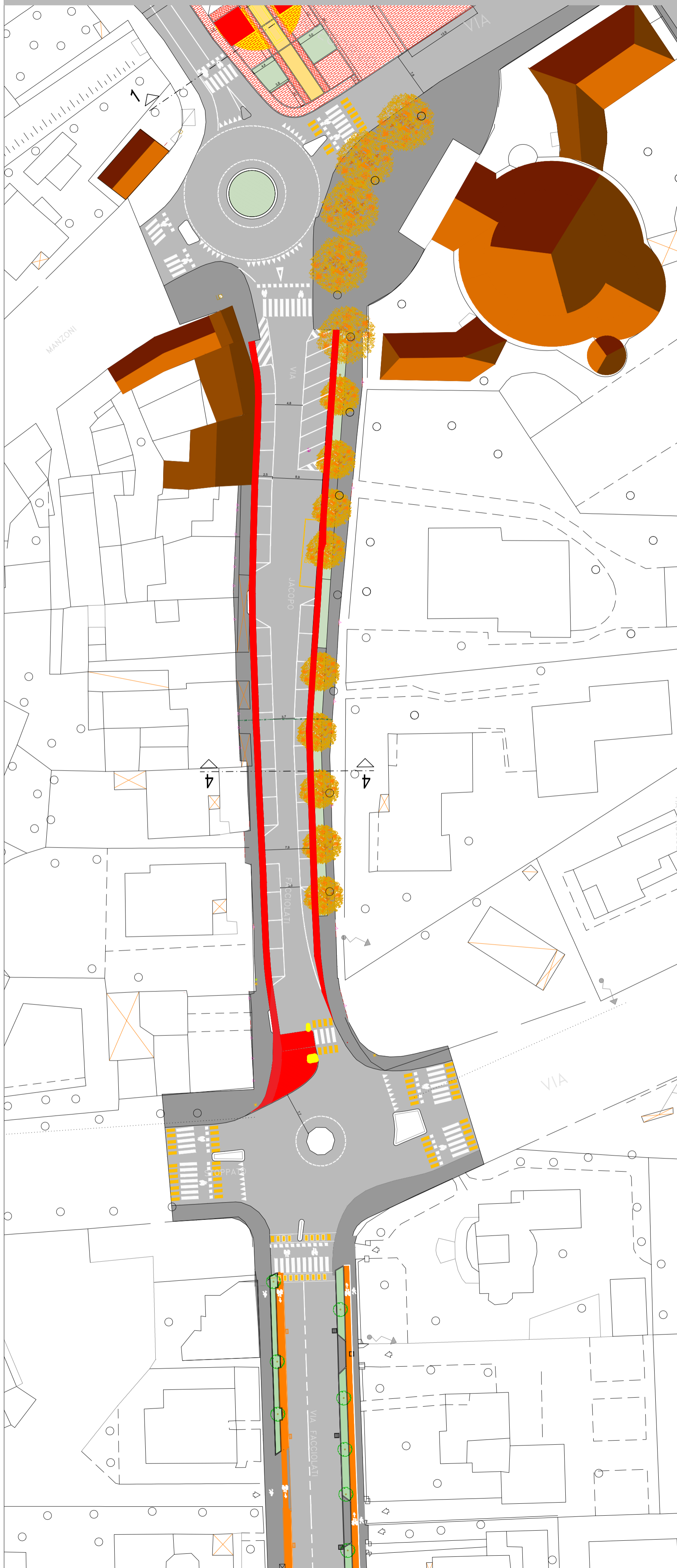
Stato di Progetto Planimetria Generale - 2° Tratto via Facciolati - Pontecorvo - scala 1:500
