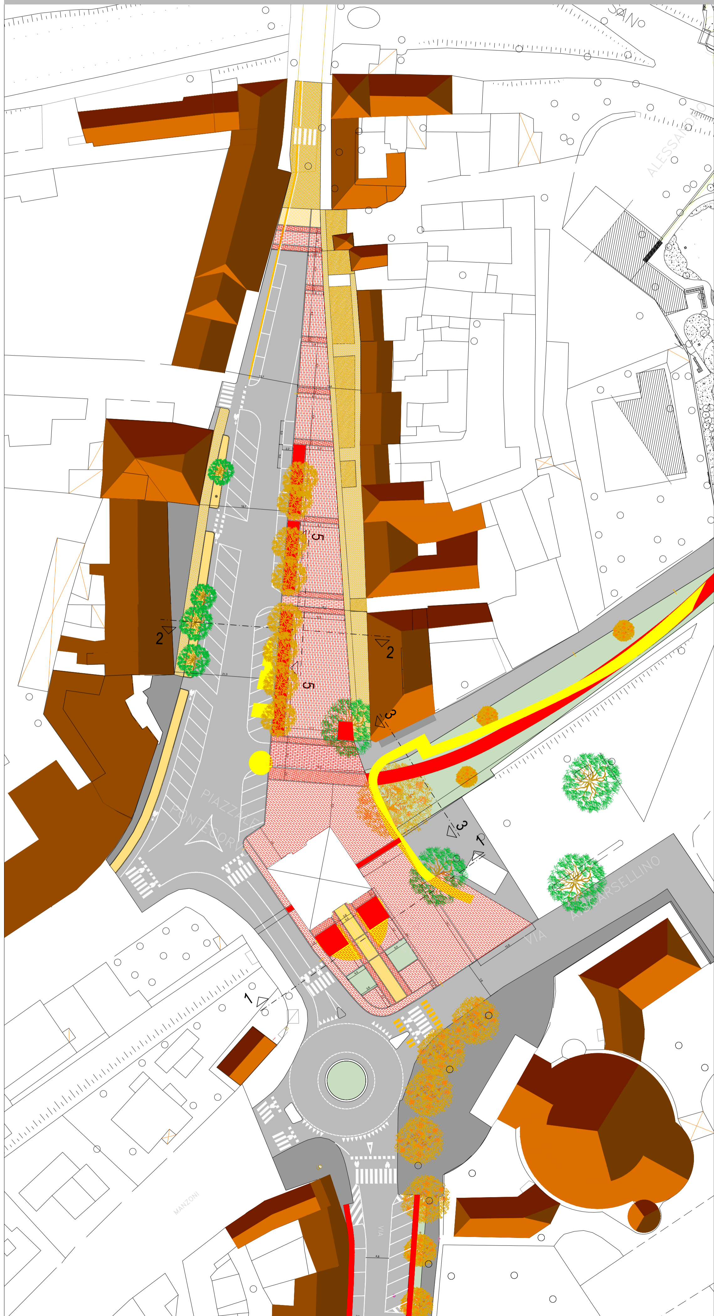
Stato di Progetto Planimetria Generale - 1° Tratto via Facciolati - Pontecorvo - scala 1:500
