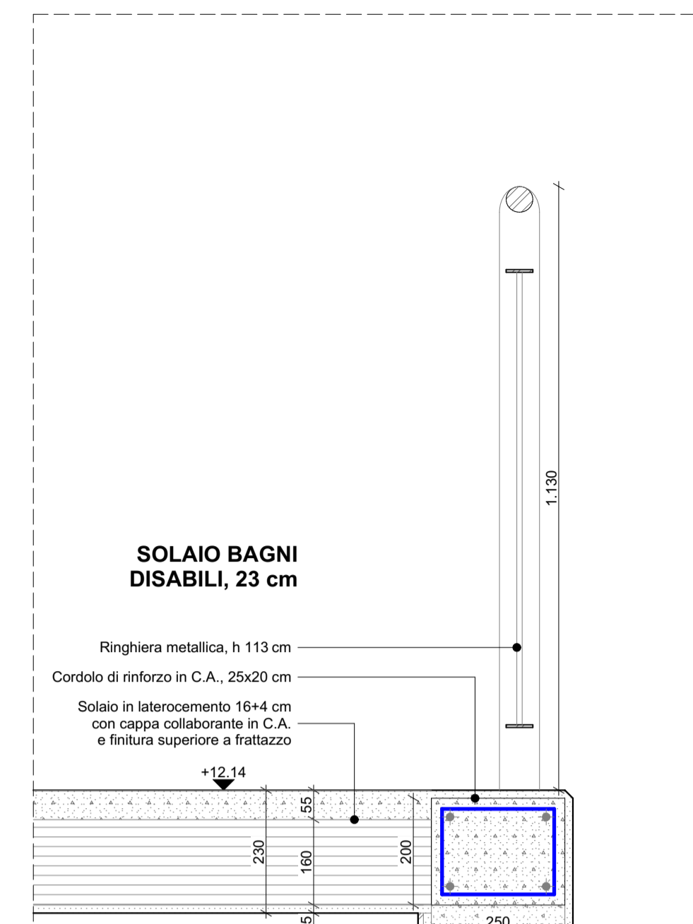
D-05 DETTAGLIO 05 1:10
