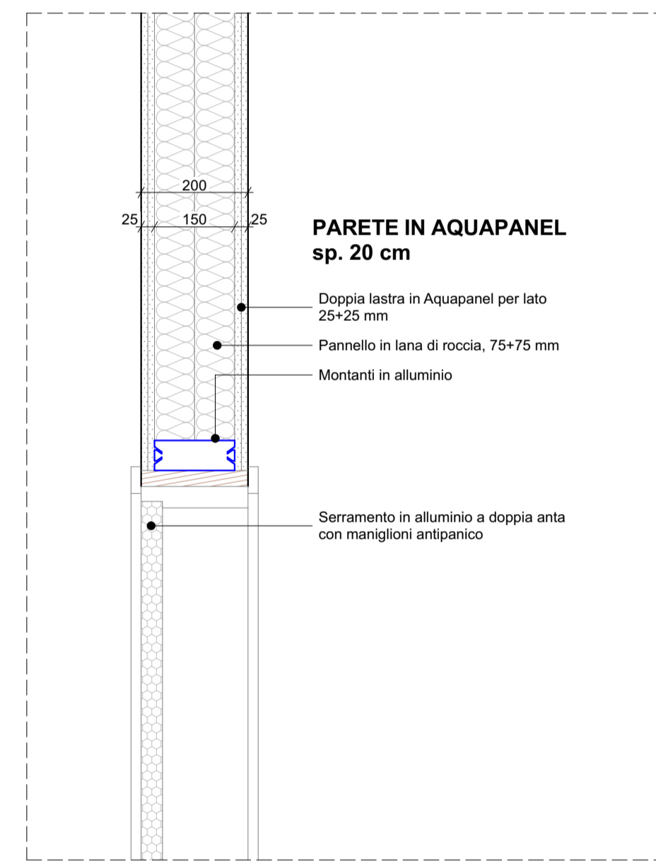
D-07 DETTAGLIO 07 1:10
