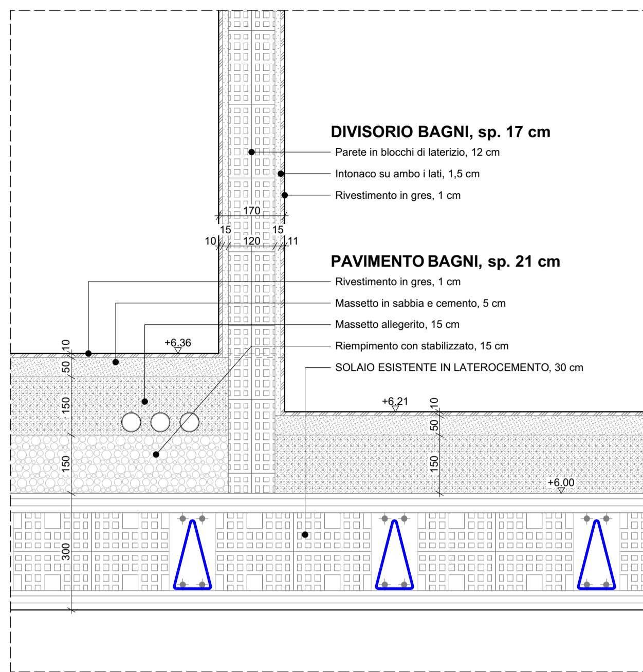
D-01 DETTAGLIO 01 1:10
