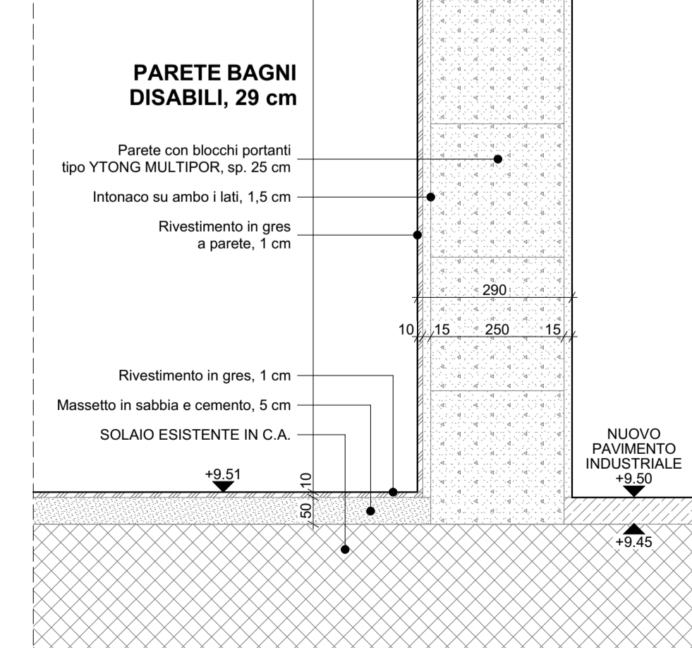
D-05 DETTAGLIO 05 1:10
