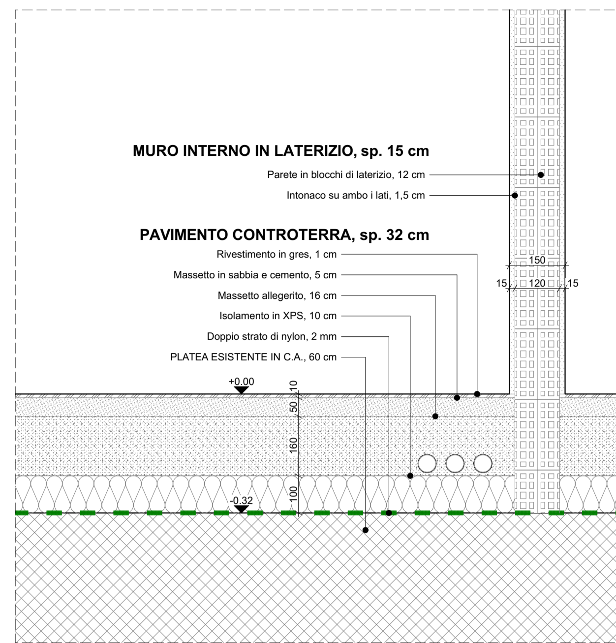
D-02 DETTAGLIO 02 1:10
