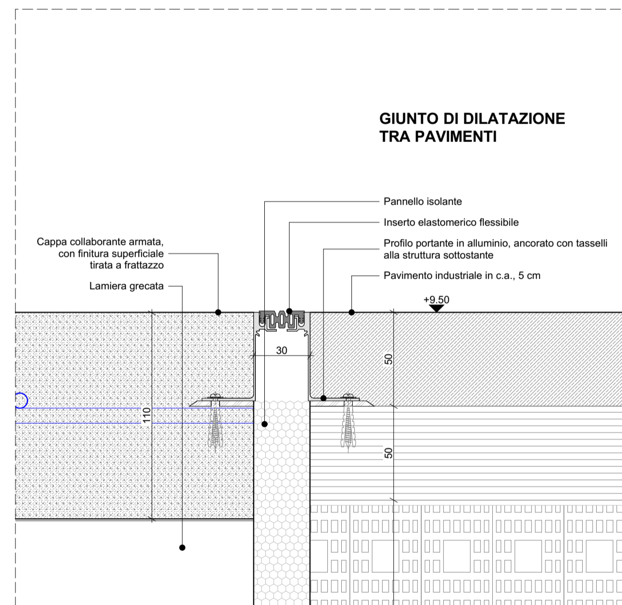
D-21 DETTAGLIO 1:2
