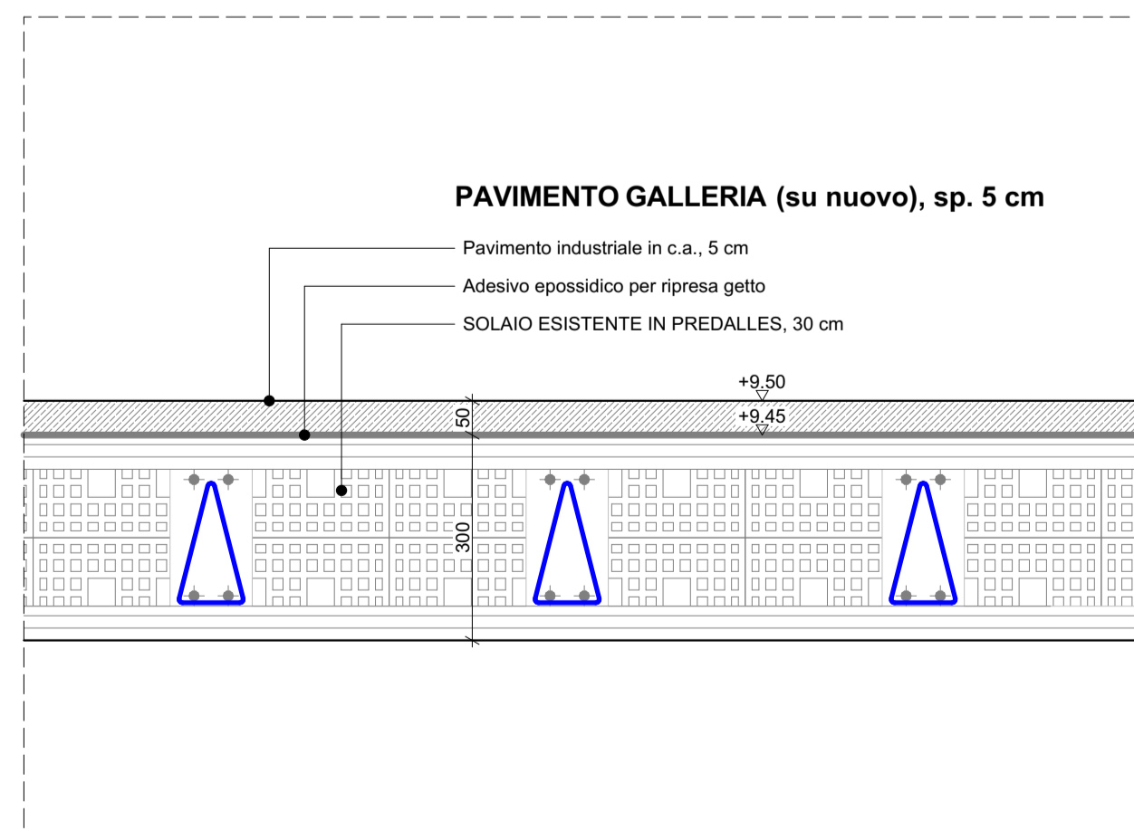
D-03 DETTAGLIO 03 1:10
