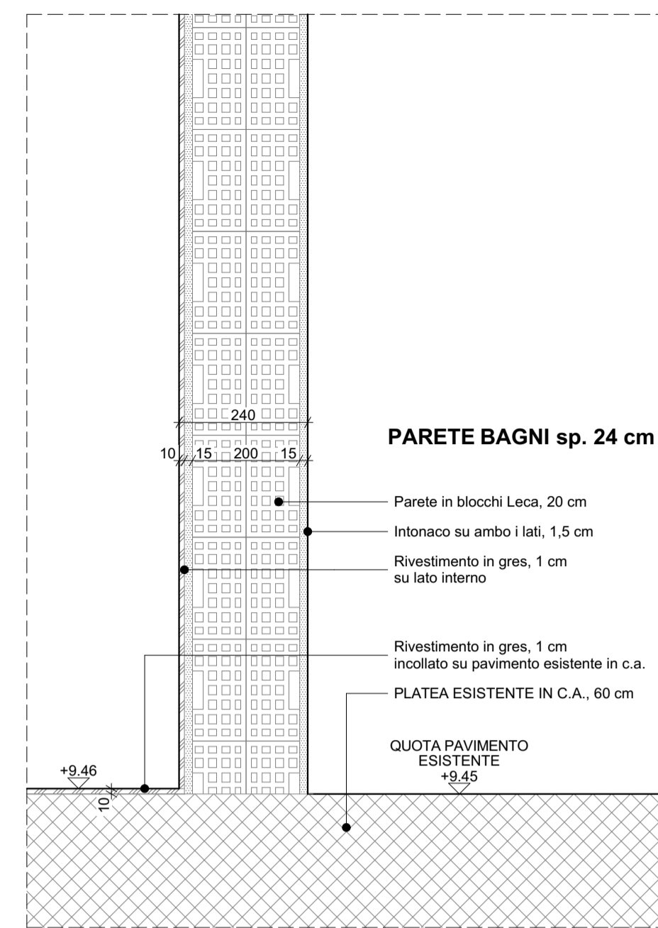
D-06 DETTAGLIO 06 1:10
