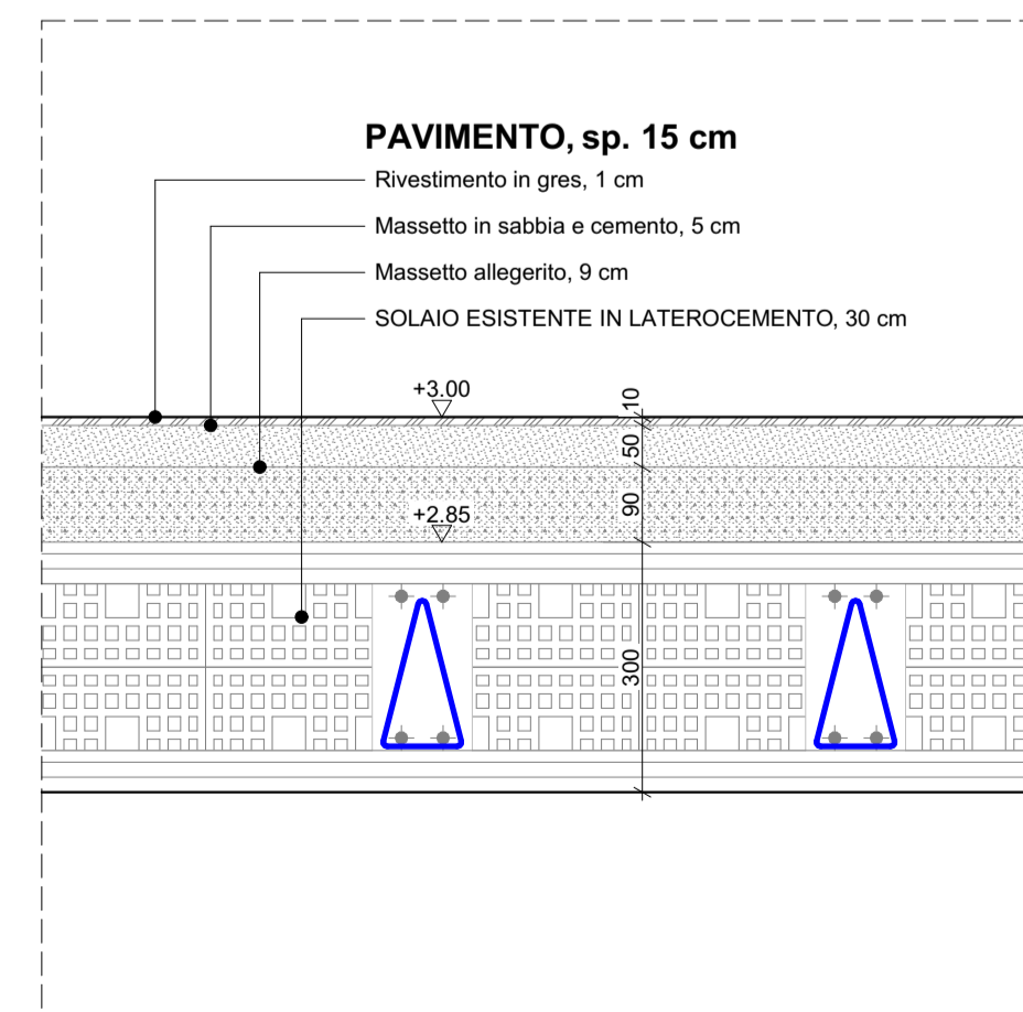
D-10 DETTAGLIO 10 1:10
