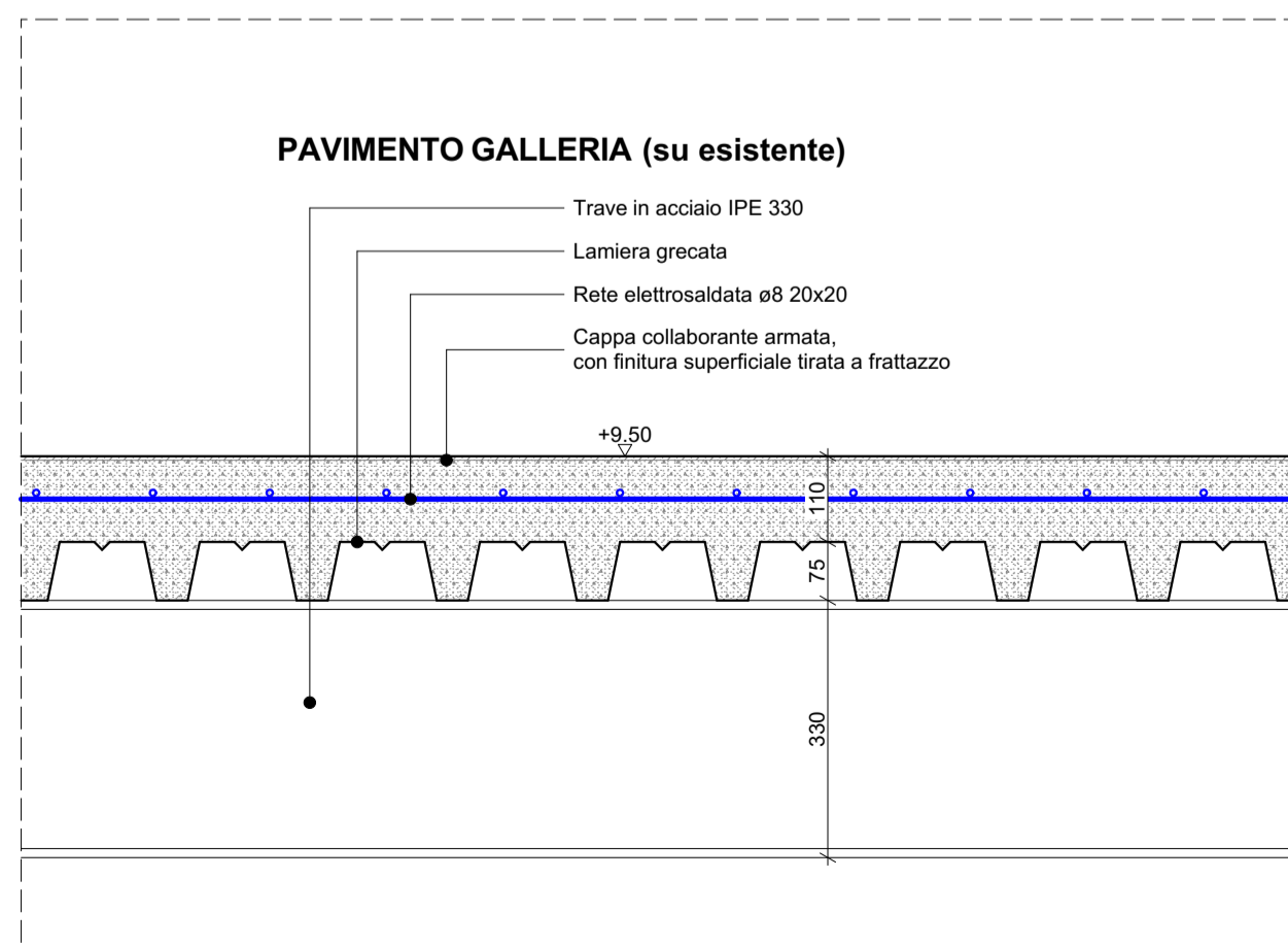
D-08 DETTAGLIO 08 1:10
