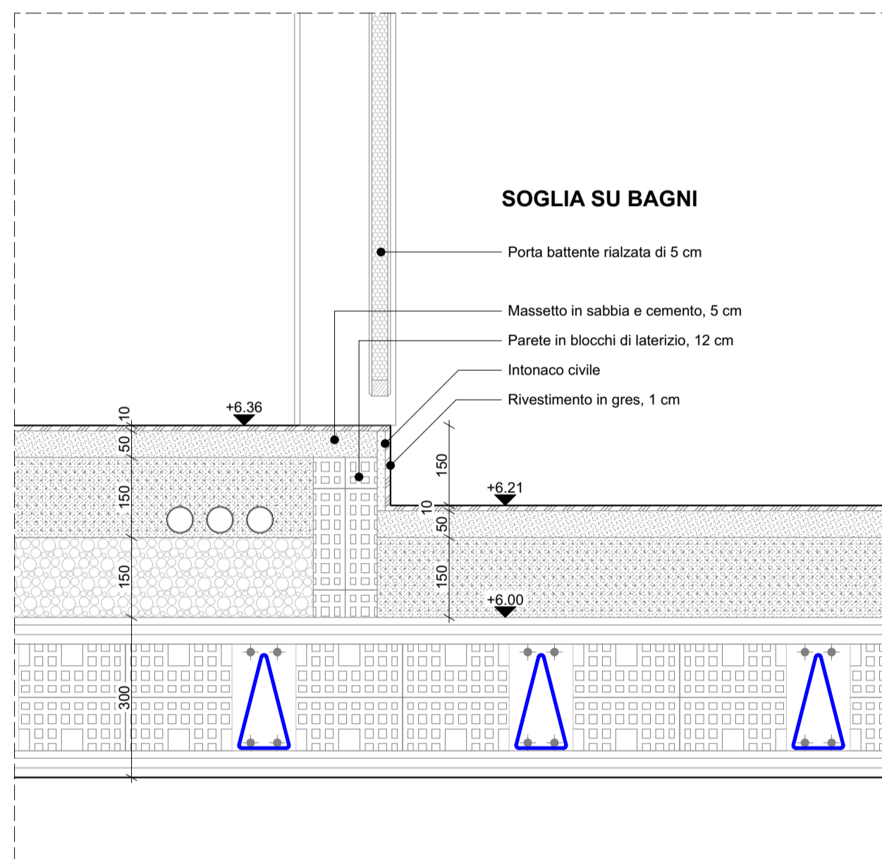
D-01 DETTAGLIO 01 1:10
