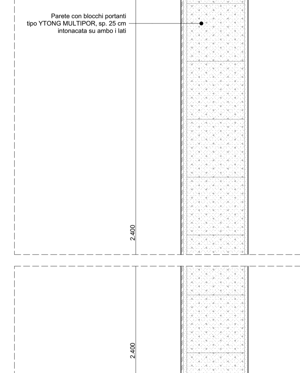
D-06 DETTAGLIO 06 1:10
