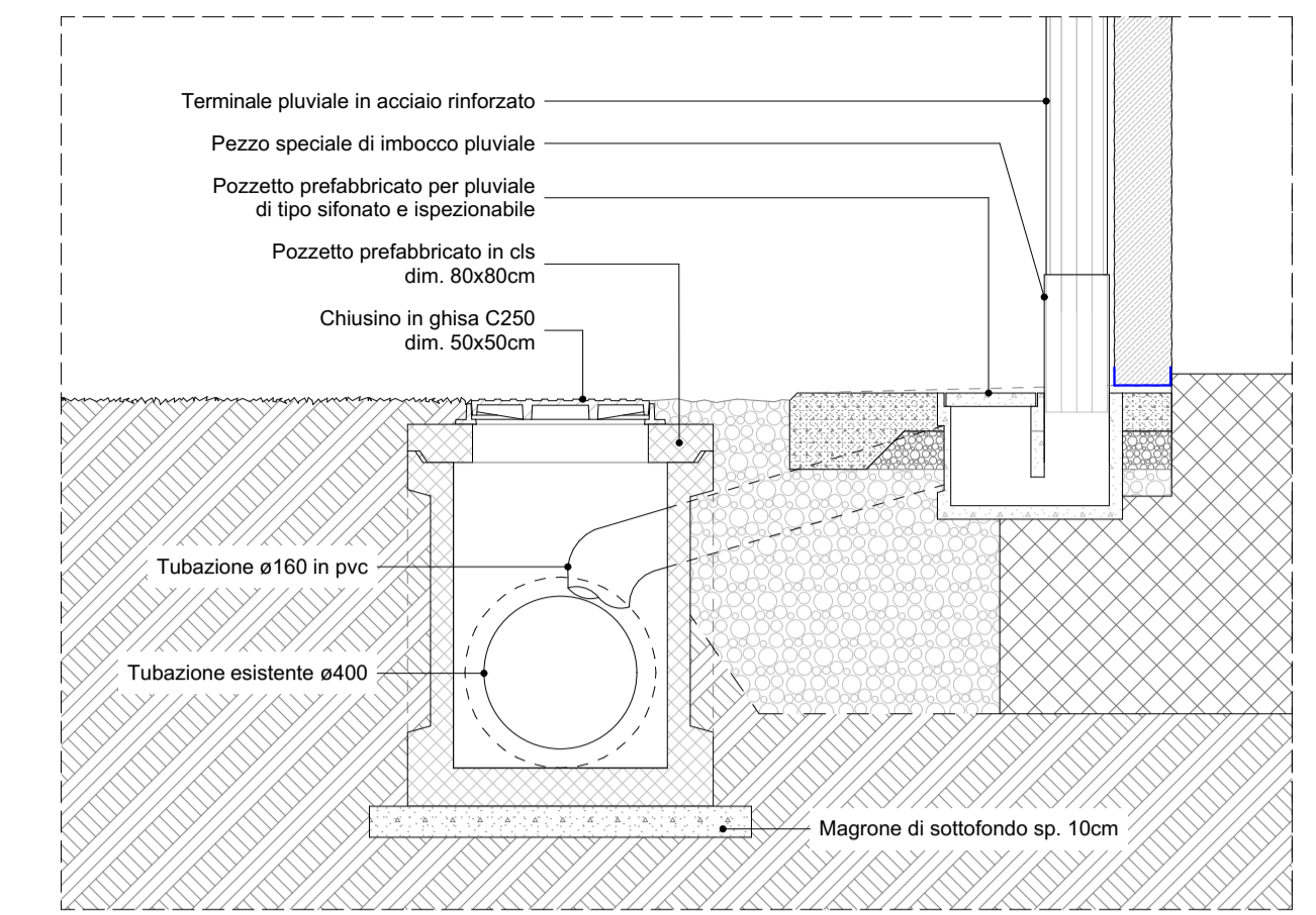
ALLACCIO LINEA ACQUE BIANCHE 1:20
