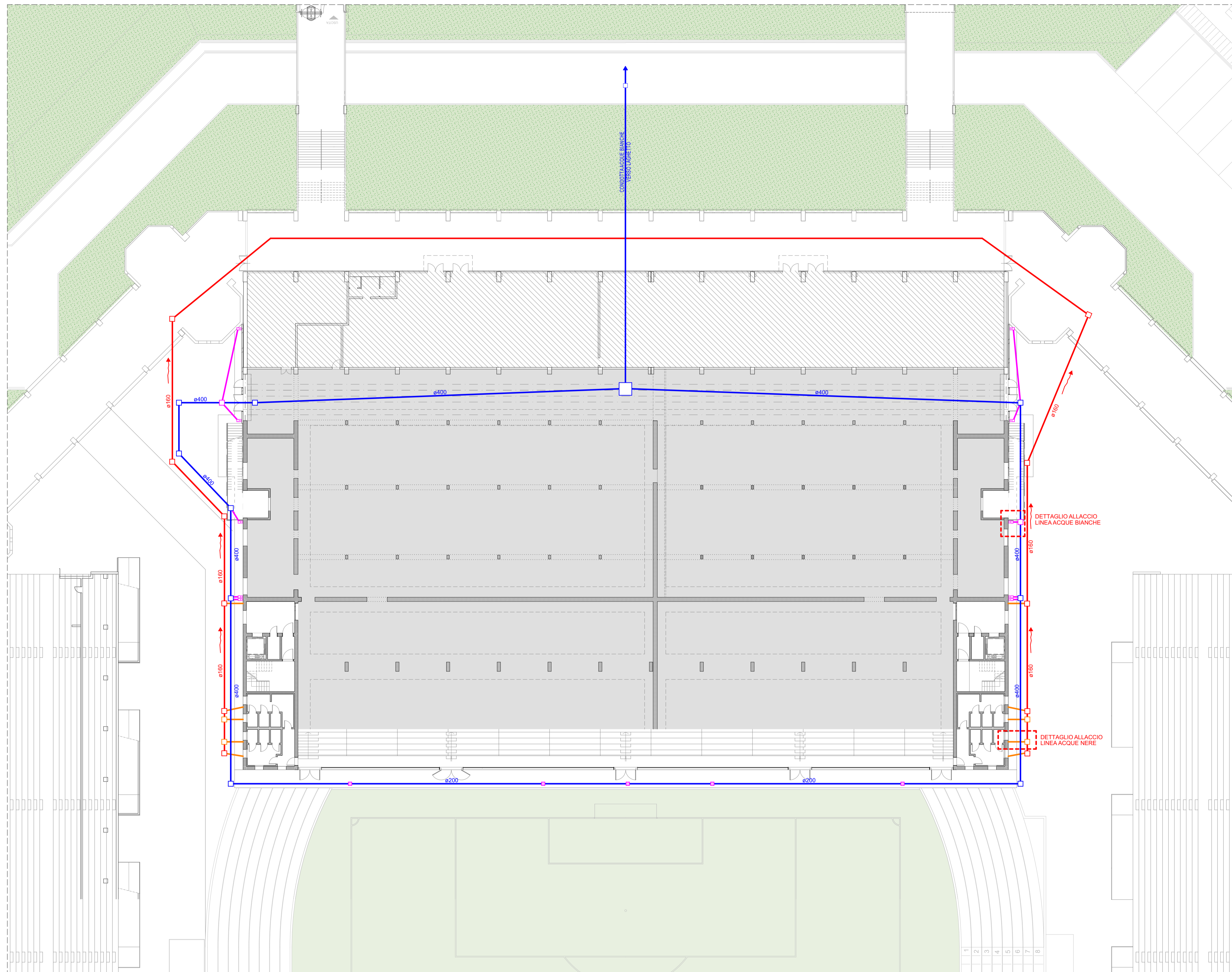
0. SCHEMA FOGNATURE 1:250
