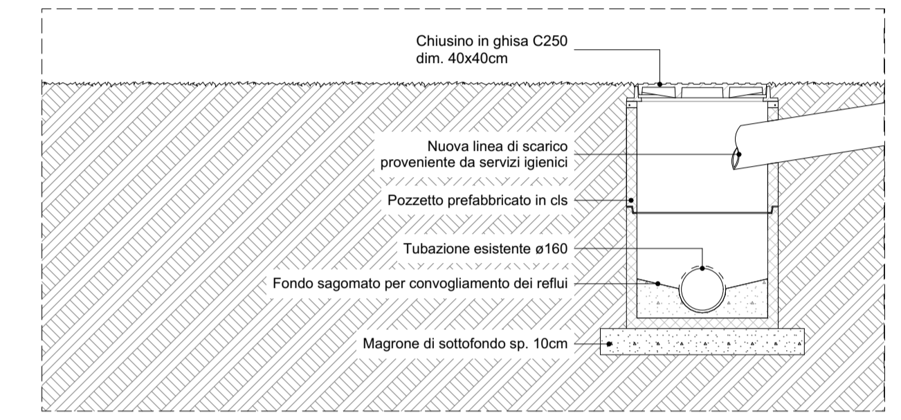
ALLACCIO LINEA ACQUE NERE 1:20
