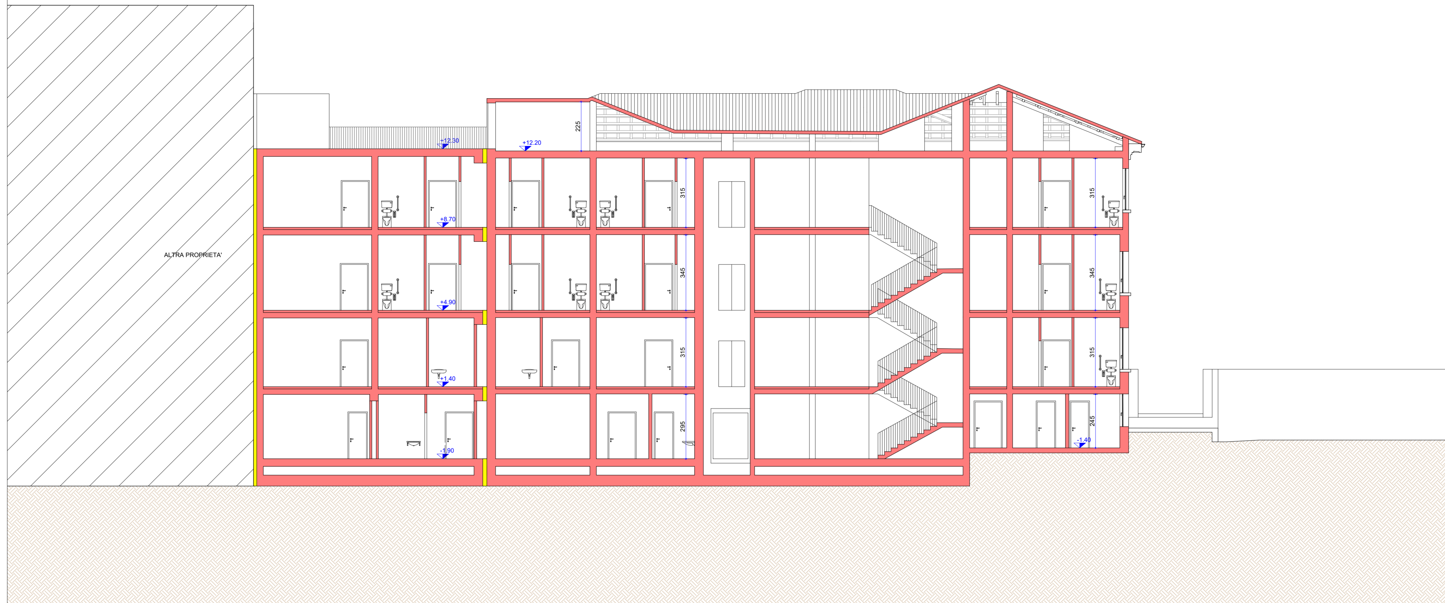
SEZIONE 3-3
