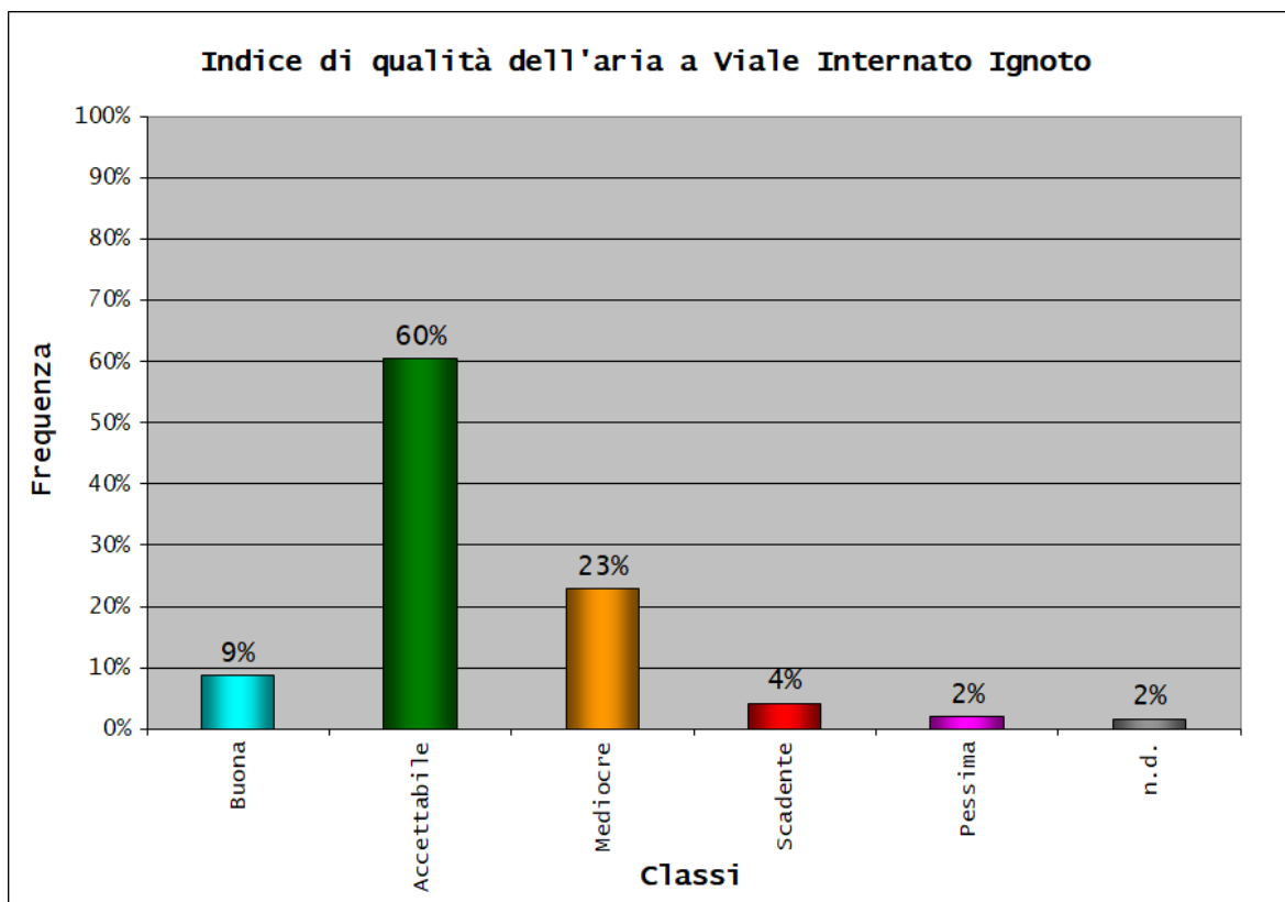
Figura 8.1: IQA 2020 a APS1
