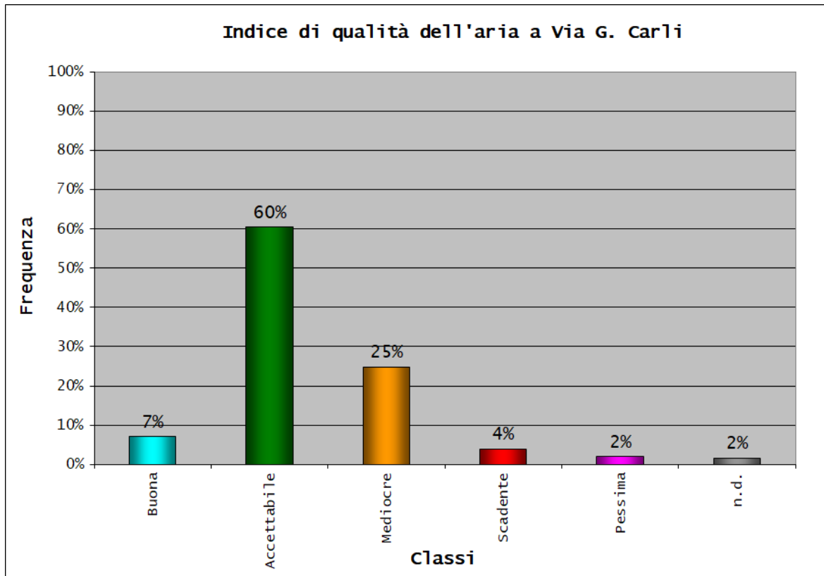
Figura 8.2: IQA 2020 a APS2
