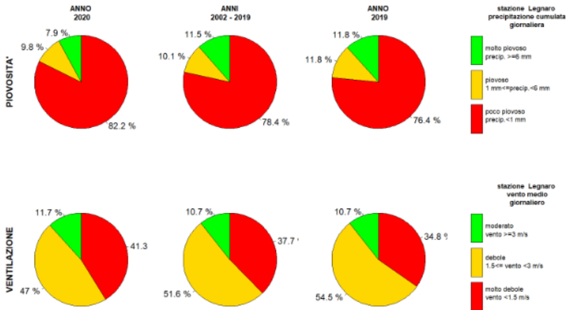
Figura 3.1: Frequenze di vento e pioggia per classi: anno 2020 a confronto con il 2019 e con la media 2002-2019
